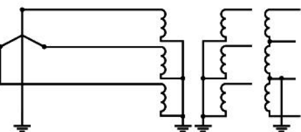
Рисунок Б.9 - Схема включения однофазных заземляемых трехобмоточных трансформаторов в трехфазных электрических сетях с заземленной нейтралью и напряжением 110 кВ и выше
