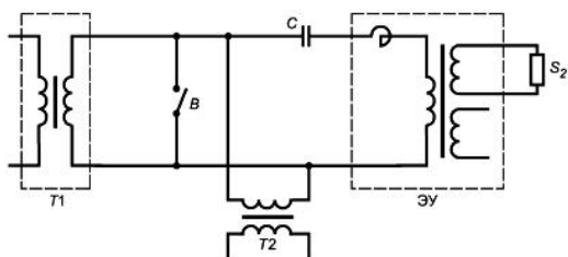
Рисунок 2 - Эквивалентная схема емкостного трансформатора
