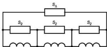
Рисунок 1 - Схема подключения фазных нагрузок
