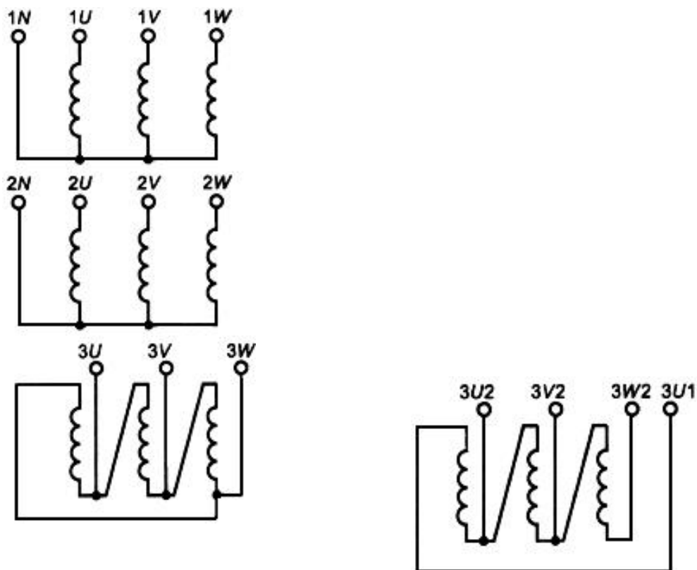
Рисунок Ж.5 - Маркировка трехфазного трансформатора ( Y_H/Y_H/D-0-5 )
