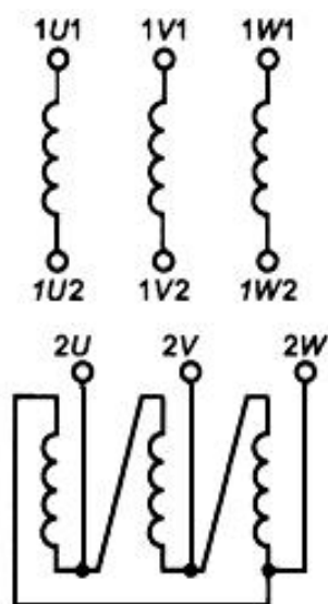
Рисунок Ж.7 - Маркировка трехфазного автотрансформатора ( Y_H авто/D -0) Рисунок Ж.8 - Маркировка линейного регулирующего трансформатора с возбуждающей обмоткой, соединенной в треугольник
