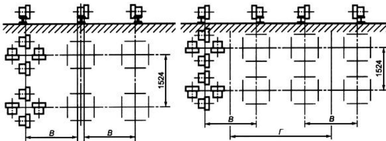
Рисунок Г.2 - Трансформаторы массой от 200 до 255 т
